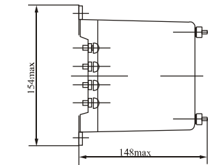
板前接线
