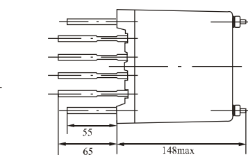
板后接线
