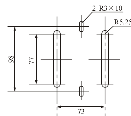
板后接线开孔
