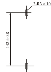
板前接线开孔
